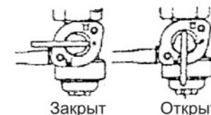
Топливный краник
